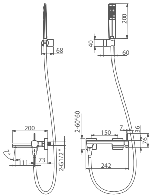
Misturadora duche/banheira monocomando.
