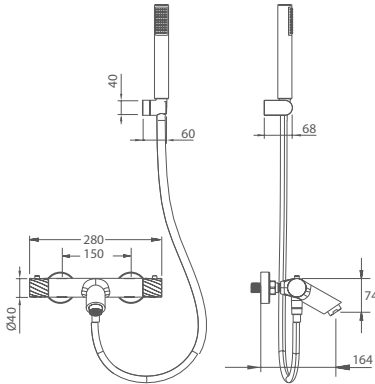
Misturadora termostática de duche/banheira.
