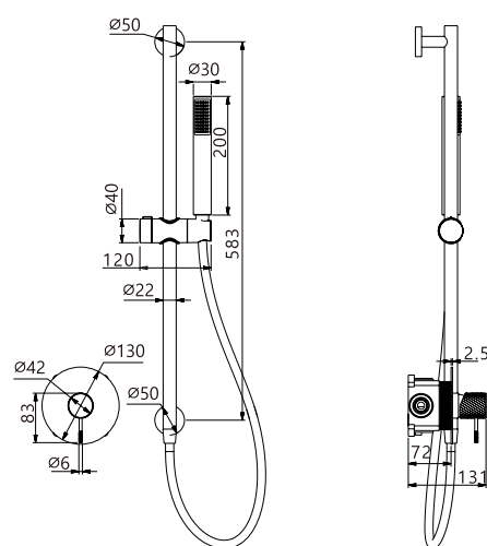
Rampa suporte para chuveiro de mão com entrada de água a parede. Suporte do chuveiro de mão regulável em altura. Chuveiro de mão de 1 posição. Torneira monocomando em latão. Caudal medio 10 l/min. Flexível de 150 cm. Cartucho monomando cerâmico Ø35 mm.
