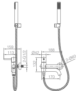
Misturadora duche/banheira monocomando.
