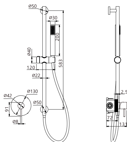
Conjunto de duche 1 via - rampa com chuveiro de mão.
