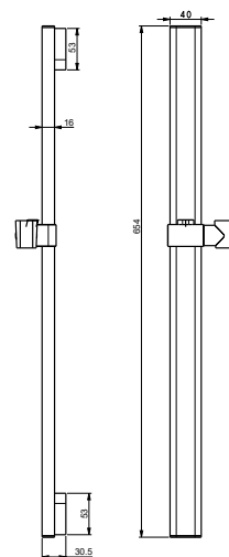
Rampa suporte para chuveiro de mão Barra de aço inox. S.304 extraplana . Suporte do chuveiro de mão regulável em altura.
